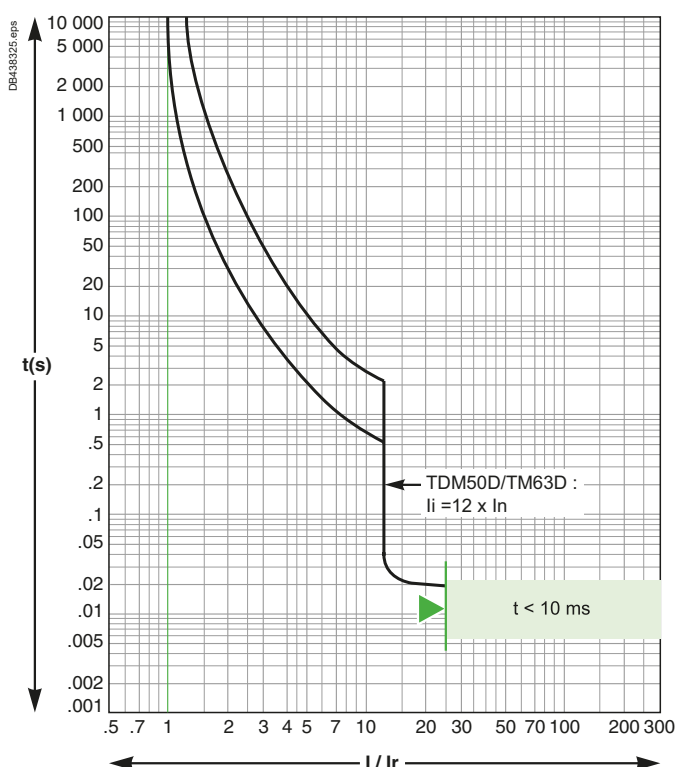
TM50D/TM63D
