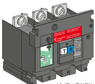
VigiPacT NSX
